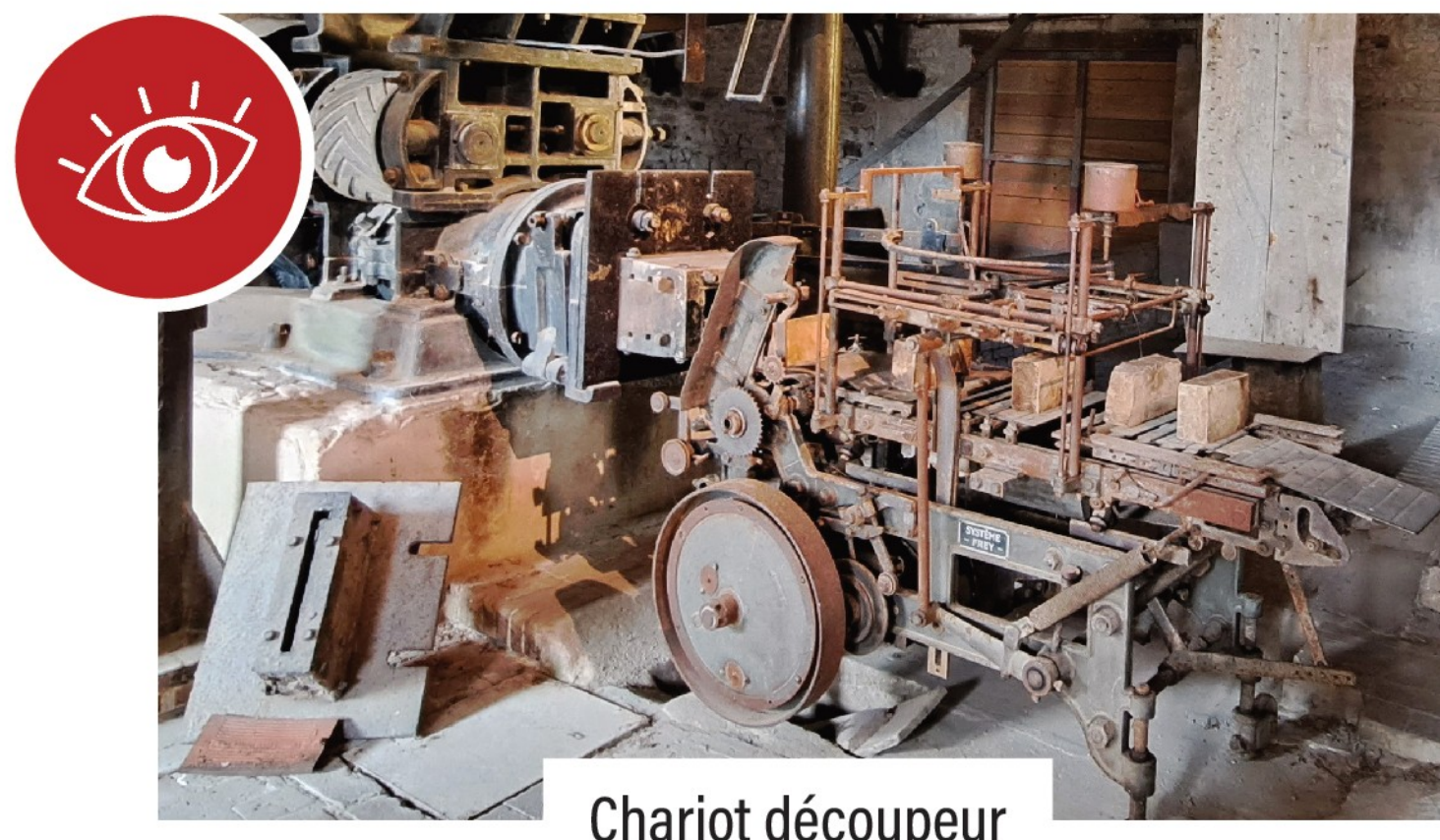
Chariot découpeur
